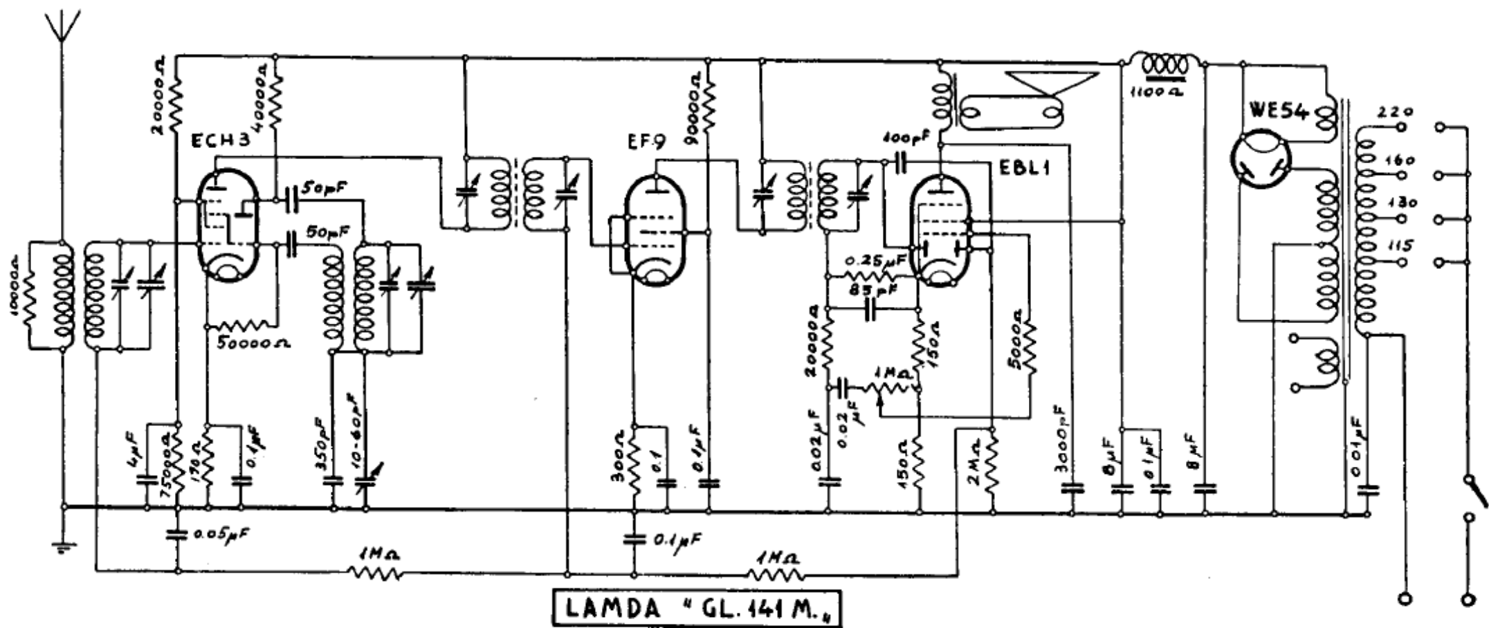
LAMDA (Olivieri e Glisenti). — Mod. « Lamda GL 141 M e R 164 M ». — Produzione 1940-1941. — Gamma: m. 500-1500 kHz. — Media frequenza: 475 kHz.
